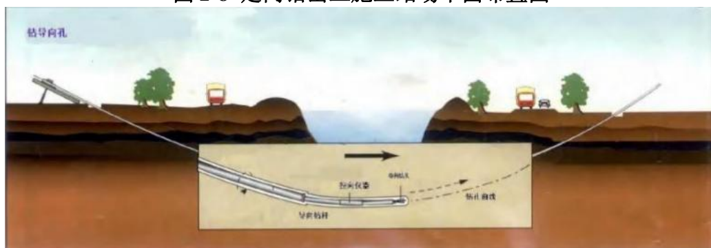
图 2-9 定向穿越管线施工示意图（钻导向孔）
