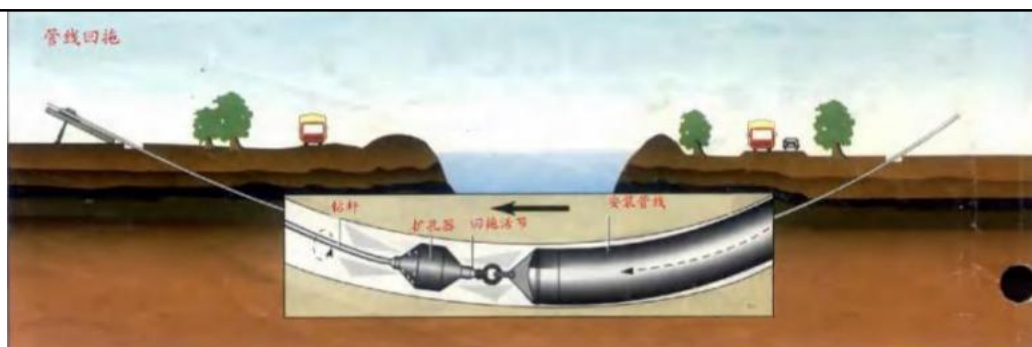
图 2-11 定向穿越管线施工示意图（回拖管线）
