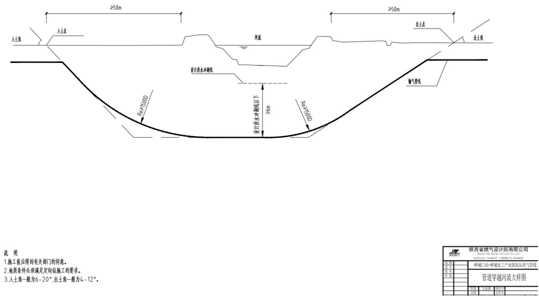
图 3-1 项目管道穿越大沙河示意图
