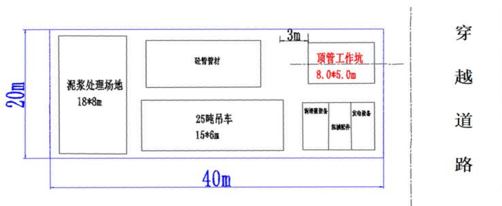
图 2-12 顶管施工场地平面布置示意图
