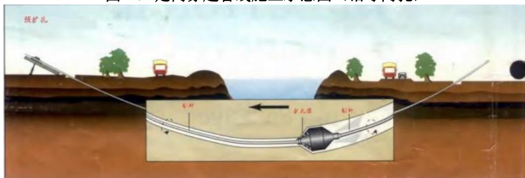
图 2-10 定向穿越管线施工示意图（扩孔）
