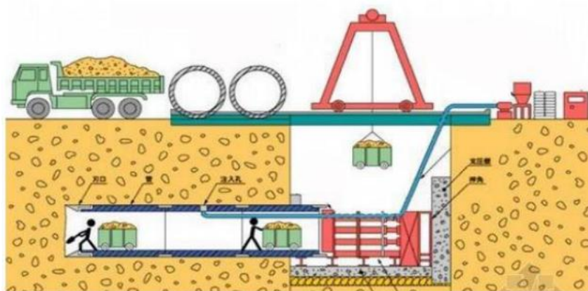
图 2-13 顶管穿越施工示意图
