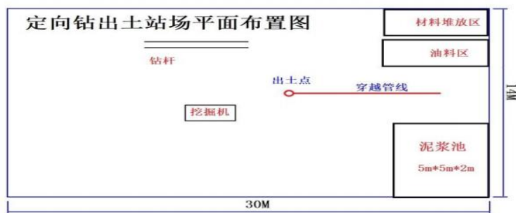
图 2-8 定向钻出土施工站场平面布置图
