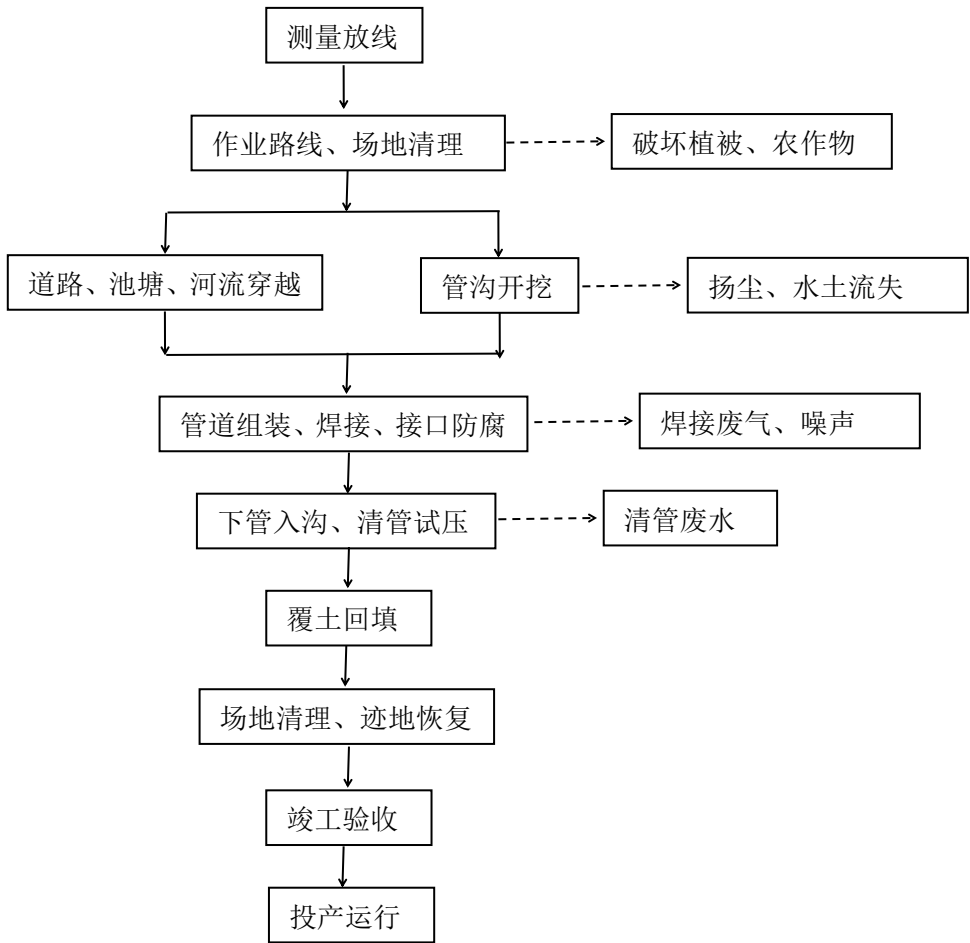
图 2-3 管线施工工艺流程及产污节点示意图
