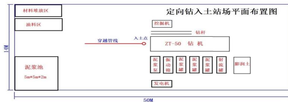
图 2-7 定向钻入土施工站场平面布置图
