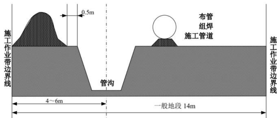
图 2-5 管沟开挖作业示意
