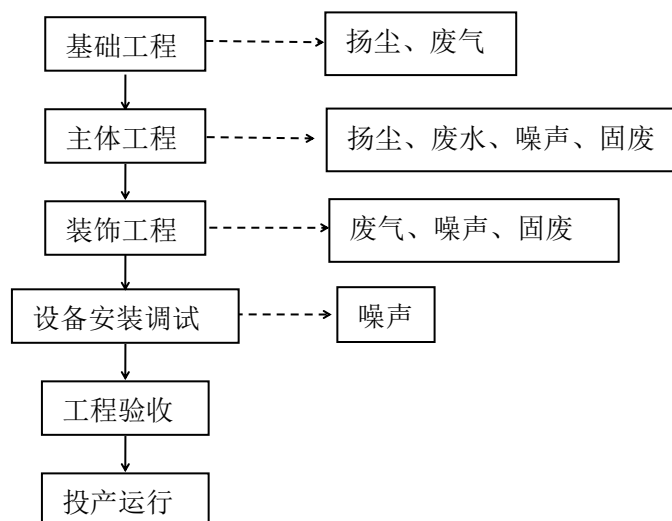
图 2-4 峰城区化工产业园调压站施工期工艺流程及产污节点示意图
