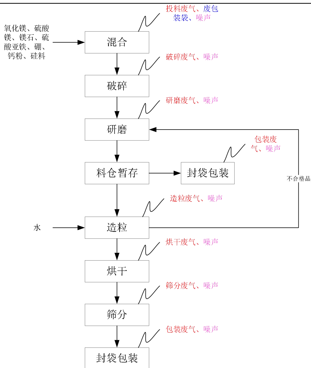
图2-3 项目生产工艺及产污环节图
